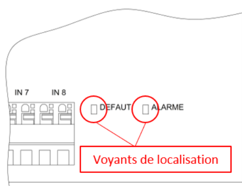
Module adressable 8 voies – ME8
