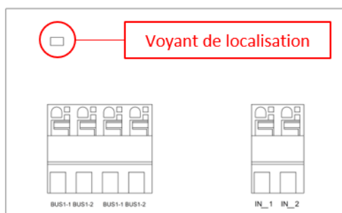
Module adressable 1 voie - ME1
